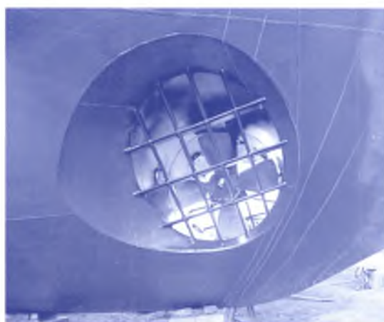
Installation d'un propulseur d'étrave sur le N.M. Lomer-Gouin pour faciliter les manœuvres d'accostage du navire
