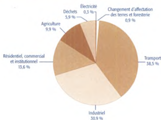
Graphique 4 : Principales sources d'émissions de gaz à effet de serre au Québec en 2002
