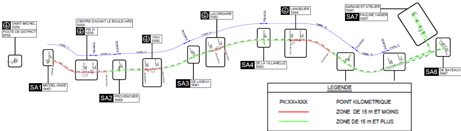
Figure 1. Profondeur du tracé du tunnel du prolongement de la ligne bleue
