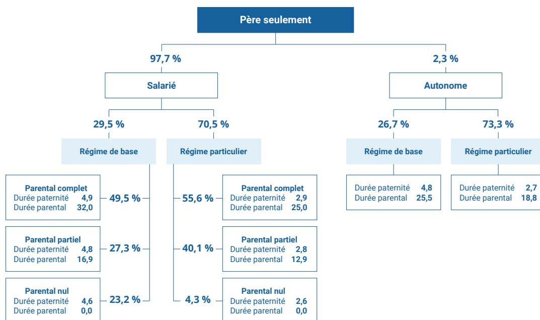
Figure 9. Choix du régime et durée des prestations (en semaines) – situation 2
