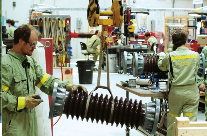
À l'atelier de remise à neuf de Madawaska, dans le Bas-Saint-Laurent, l'électricien d'appareillage Yves Olivier Ménard inspecte la colonne support d'un disjoncteur.
